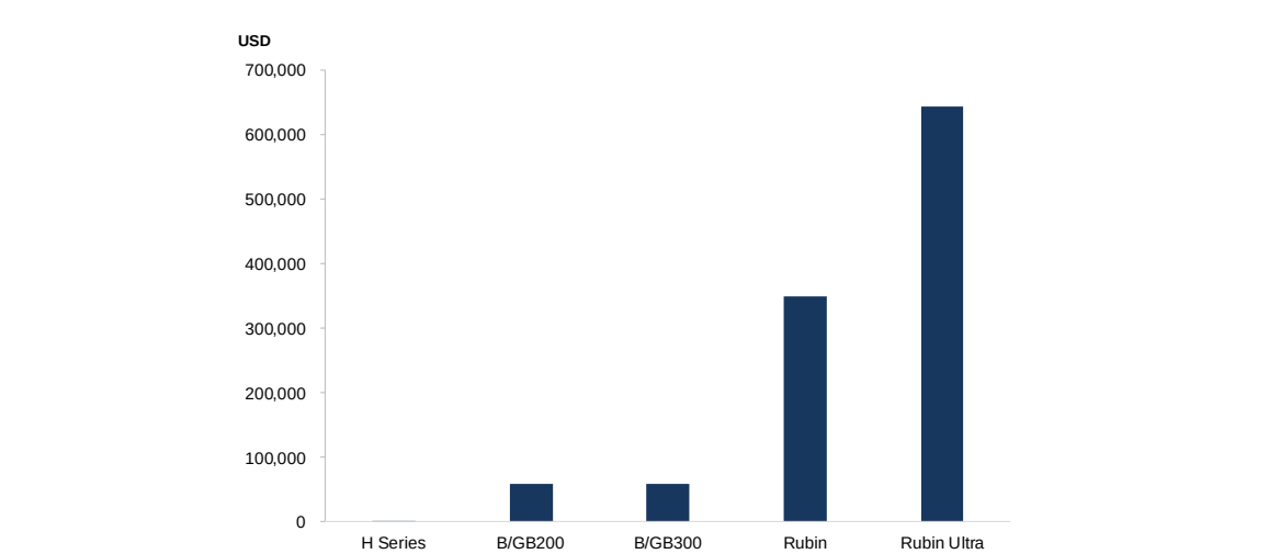
圖 7：Power Content Value 隨 Rubin/Rubin Ultra Power rack/HVDC 導入大幅提升
