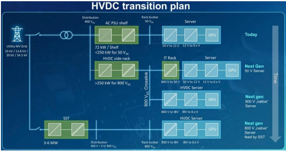
圖 8：電源架構趨勢明確，產值持續提升。台達電擁電網-電力傳輸-伺服器至板上電力解決產品
